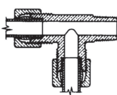
8B TEE
